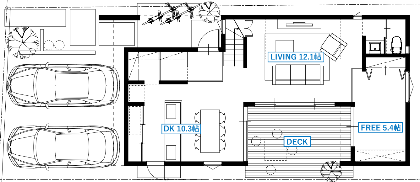
1階平面図
