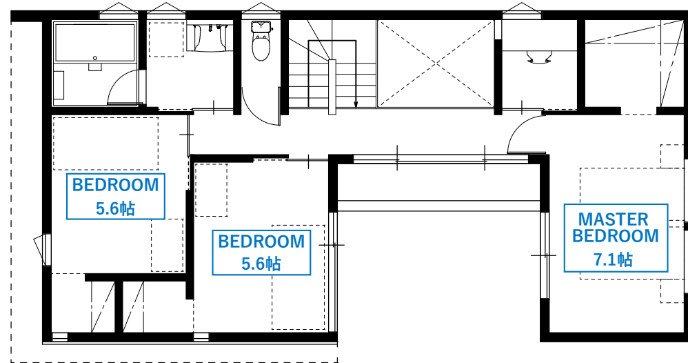
2階平面図
