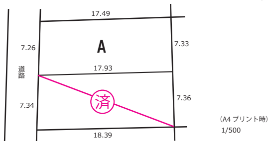
【区画図】
